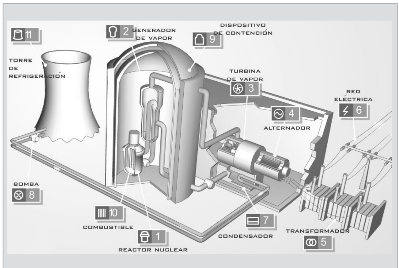
Producción de energía a través de un reactor nuclear.
